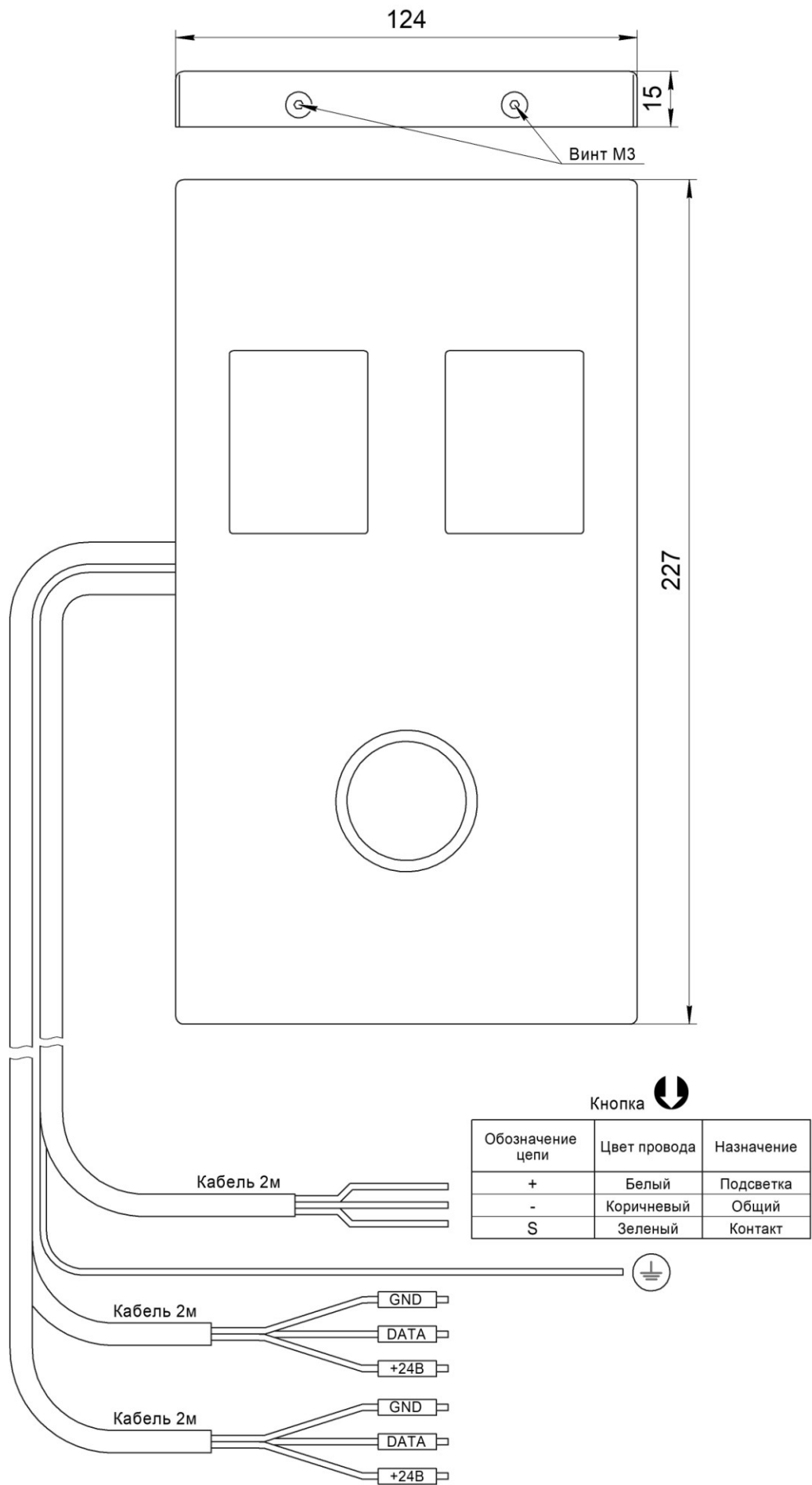
Рис.1 Внешний вид, габаритные и установочные размеры Вызывного поста КВАДРО НШЕК.468381.067
